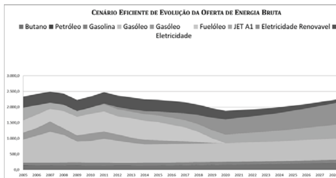
Figura 15 – Evolução da Oferta de Energia Bruta no Cenário de Eficiência em Cabo Verde
