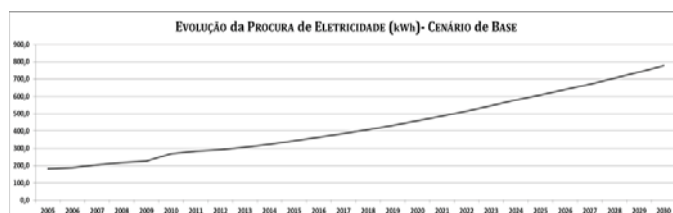
Figura 8 – Evolução da Procura Total de Eletricidade em Cabo Verde até 2030
