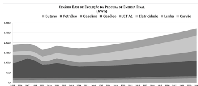
Figura 8 – Evolução da Procura Total de Energia Final para Cabo Verde até 2030
