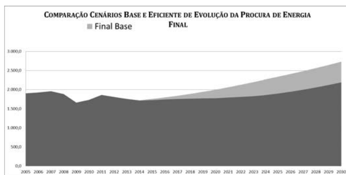
Figura 13 – Comparação da Procura de Energia Final no Cenário de Base e no de Eficiência em Cabo Verde
